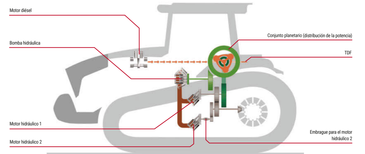
Diagrama del diseño del Fendt VarioDrive
